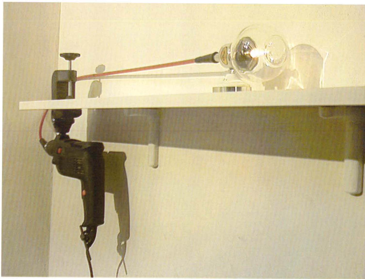
E LUCE FU 6v 120 x 20 x 40 cm circa trapano, dinamo, lampadina da 6 volt, corrente elettrica
